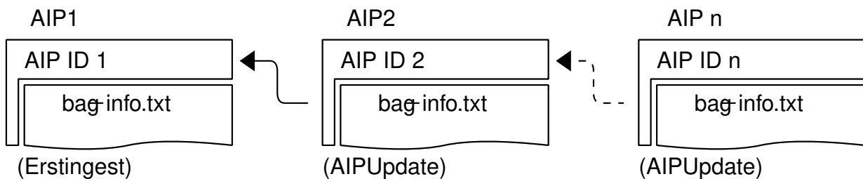
Abbildung 6. Versionsgraph
